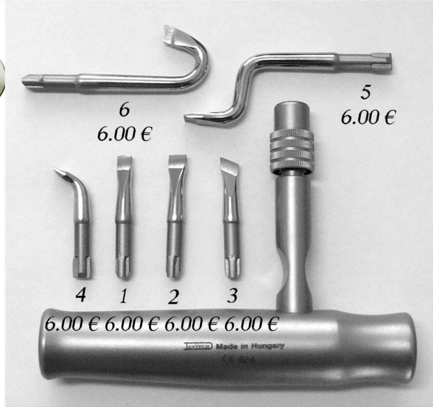
DP 1779 INSTRUMENT INDEPARTATOR LUCRARI PROTETICE TIP DENTECH ( 6 CAPETE ) KRONENENTFERNER MIT 6 EINSATZEN CROWN REMOVERS WITH 6 INSERT 84.50 €
